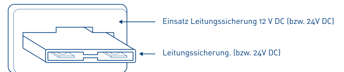
ABBILDUNG 5: SICHERUNG DER GLEICHSPANNUNGSLEITUNG 12 V DC (BZW. 24V DC)
