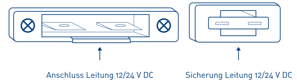
ABBILDUNG 2: STECKER FÜR DEN ANSCHLUSS MIT 12/24V DC- GLEICHSPANNUNG FÜR KOALA FOODSERVICE MIT INTEGRIERTEM KÜHLAGGREGAT ODER MIT EXTERNEM STATISCHEM KÜHLAGGREGAT.
