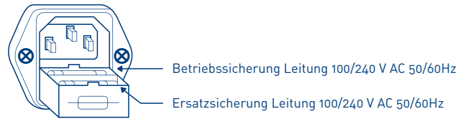
ABBILDUNG 6: LEITUNGSSICHERUNG AN WECHSELSPANNUNG 100/240 V AC 50/60Hz
