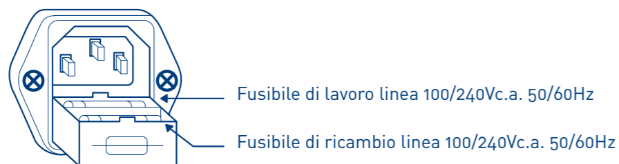
Disegno 6: FUSIBILE LINEA IN TENSIONE ALTERNATA 100/240Vc.a. 50/60Hz
