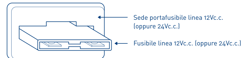
Disegno 5: FUSIBILE LINEA IN TENSIONE CONTINUA 12Vc.c. (OPPURE 24Vc.c.)
