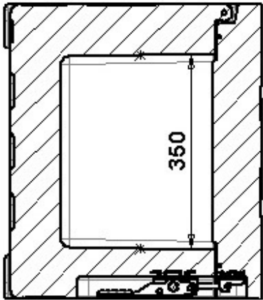
SEZIONE B-B
