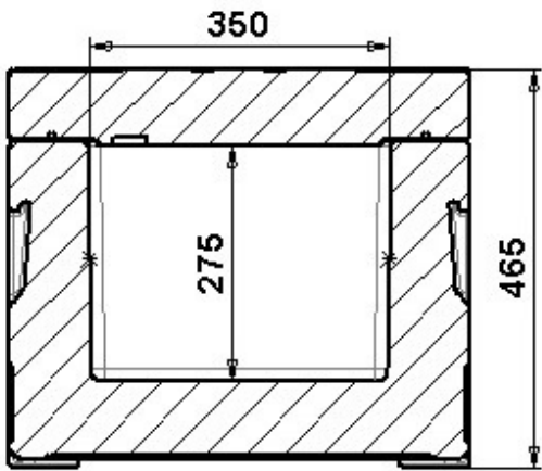
SEZIONE A-A
