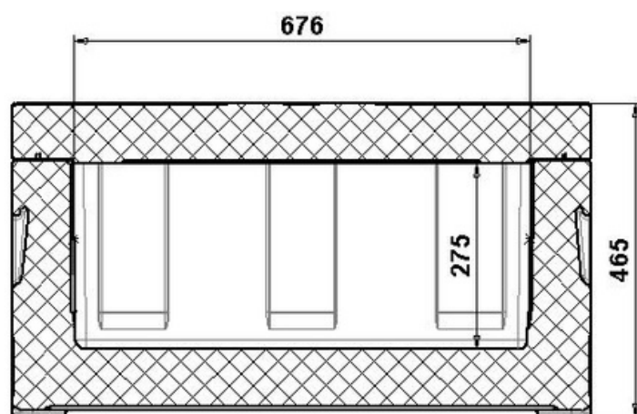
SEZIONE A-A
