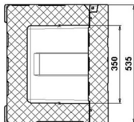
SEZIONE B-B
