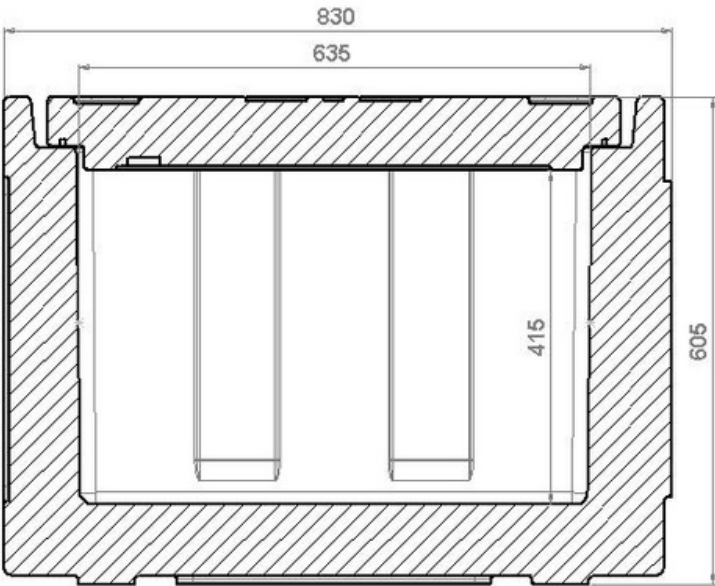
SEZIONE A-A
