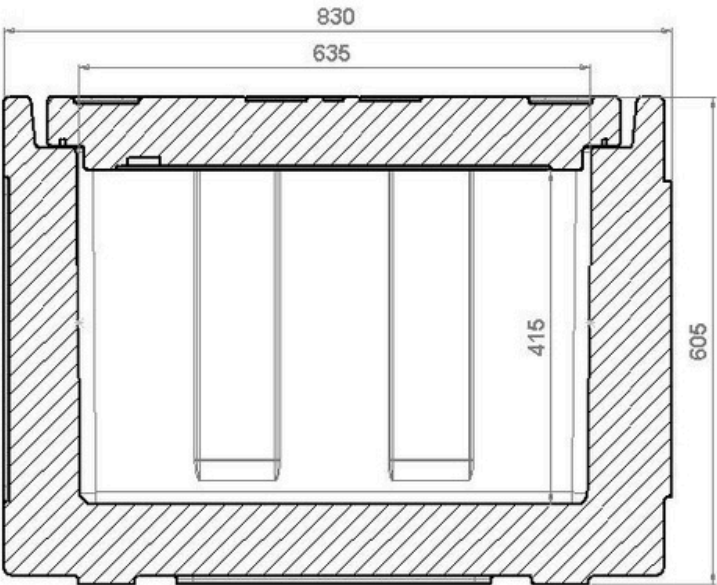
SEZIONE A-A
