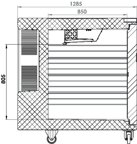
Koala 495 ventilé
