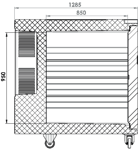
Koala 495 statique
