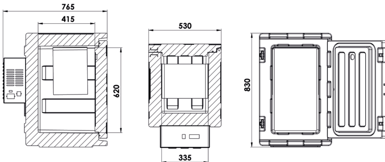
KOALA 90-XTRA GRUPPO FRIGO DORSO
