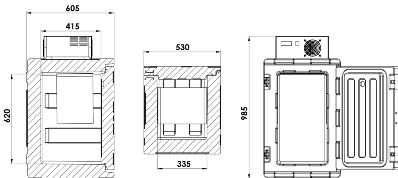
KOALA 90-XTRA GRUPPO FRIGO TETTO
