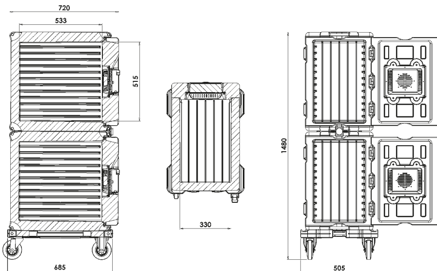
Système modulaire AF12 / KOALA90 chaud/surgelé
