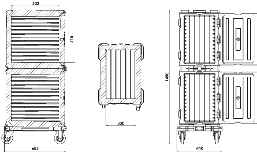
Système modulaire AF12 frais/frais
