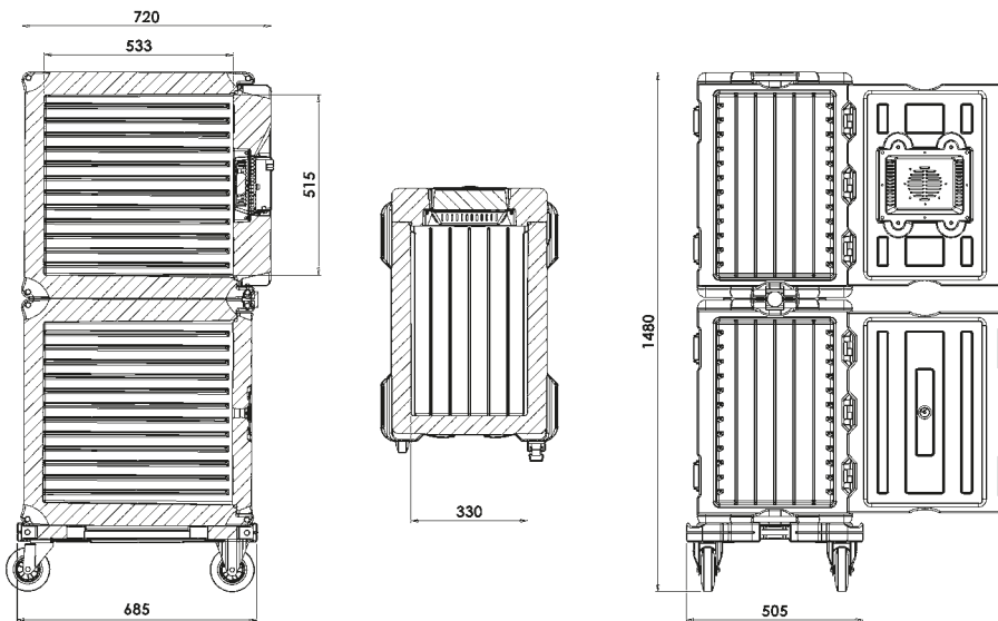
Système modulaire AF12 frais/chaud
